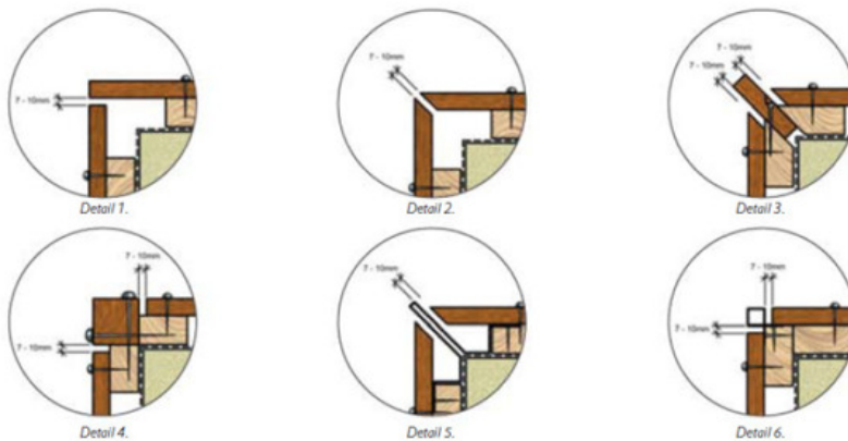
Voorbeelddetails binnenhoeken
