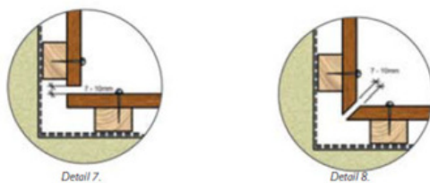
Voorbeelddetails binnenhoeken
