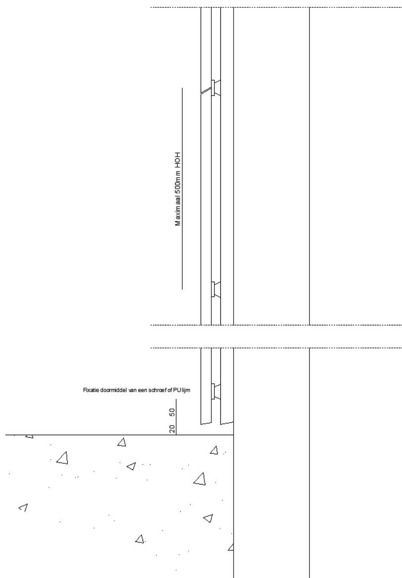
Verticale gevel (Afbeelding 2)
